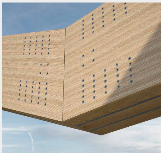
^ Trdi kolenast spoj z dvojno notranjo ploščo (LVL).
