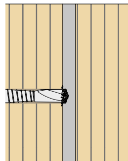
Ostružki, ki med vrtanjem zamašijo luknje v jeklu (distančniki niso nameščeni).
