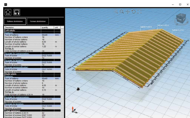
Tetőlécek kalkulációja.
