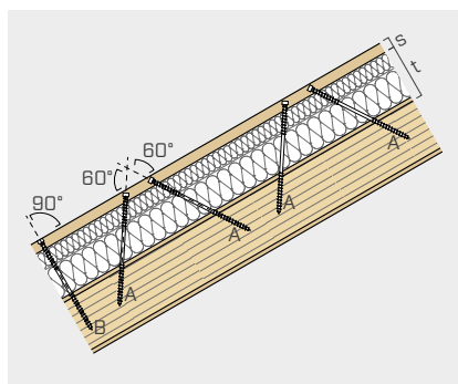
MJUK ISOLERING TÄCKNING \sigma_{(10\%)} < 50 \text{ kPa} (EN826)
