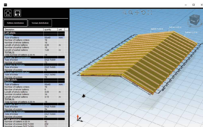
Beräkning av täcklister.
