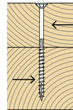
負荷と木目の角度 \alpha = 90^\circ
