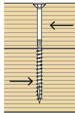
負荷と木目の角度 \alpha = 0^\circ
