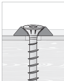
IT Rondella svasata HUS EN HUS countersunk washer DE Versenkte Unterlegscheibe HUS ES Arandela avellanada HUS FR Rondelle fraisée HUS PT Anilha de embeber HUS RU Шайба с фаской HUS
