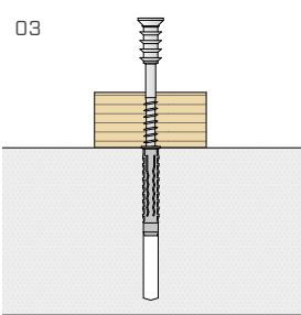
定位 DRT 螺钉。
