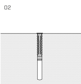
将 NDK GL 尼龙膨胀螺栓嵌入支架中。
