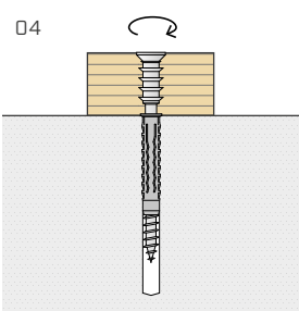
通过拧紧螺钉而固定板条，使头部与木构件齐平。
