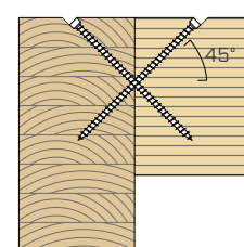
nárys
