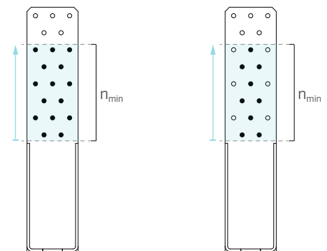
WHT20: Teilausnagelung jeweils in der Wide-Pattern- bzw. Narrow-Pattern-Konfiguration mit Montage der Mindestanzahl an Verbindern n_{\min} .
