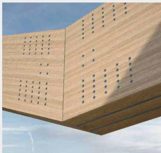
Trevägsförband med dubbel intern platta (LVL).
