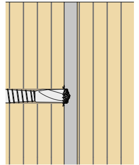
드릴링 도중에 강재의 홀을 막는 대패톱밥(스페이스 미설치)
