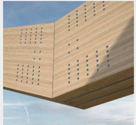
Starre knieverbinding met dubbele interne plaat (LVL).
