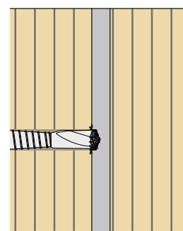
Schilfers blokkeren de gaten in het staal tijdens het boren (afstandhouders niet geïnstalleerd).
